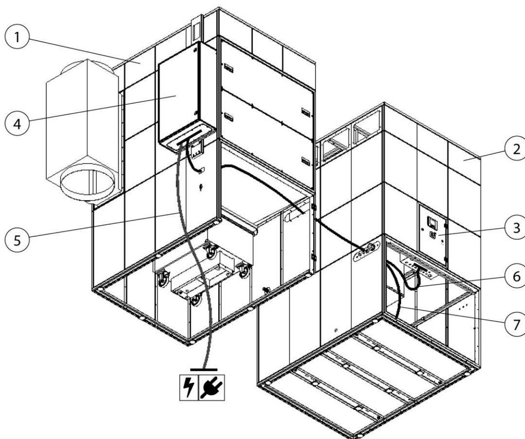
Bild 33: Exempel: Kabeldragning för sugprestandareglering
