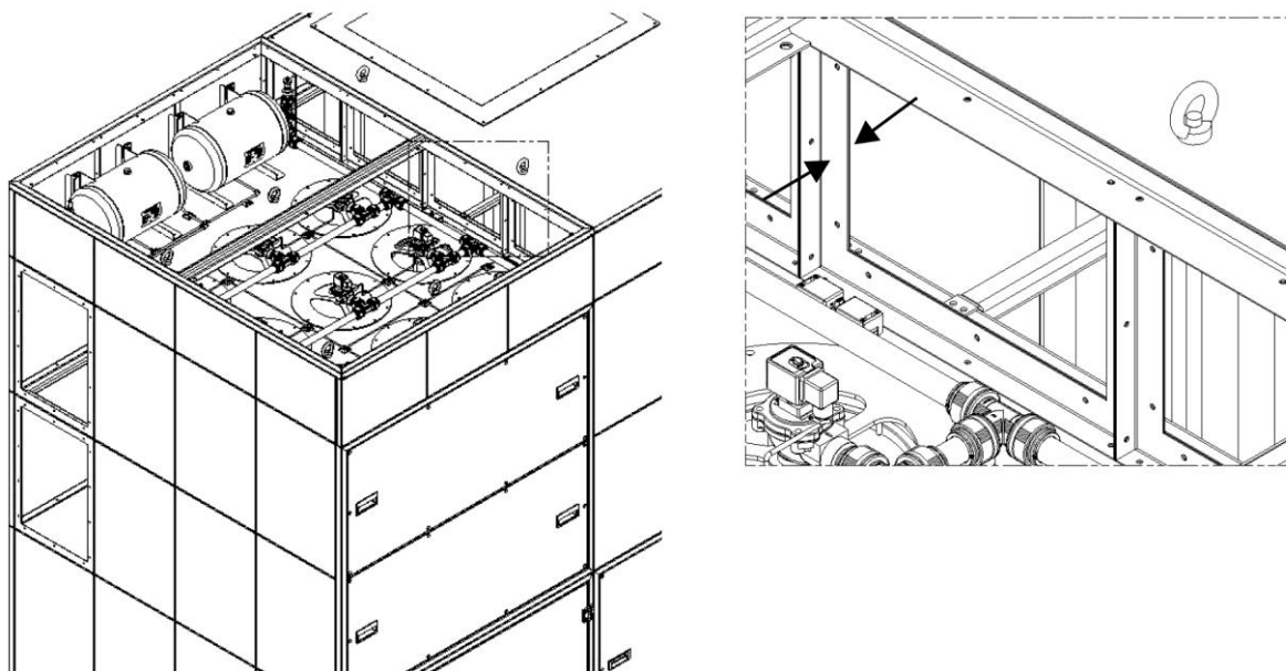
Bild 21: Ansluta fläkt delen till filterdelen
