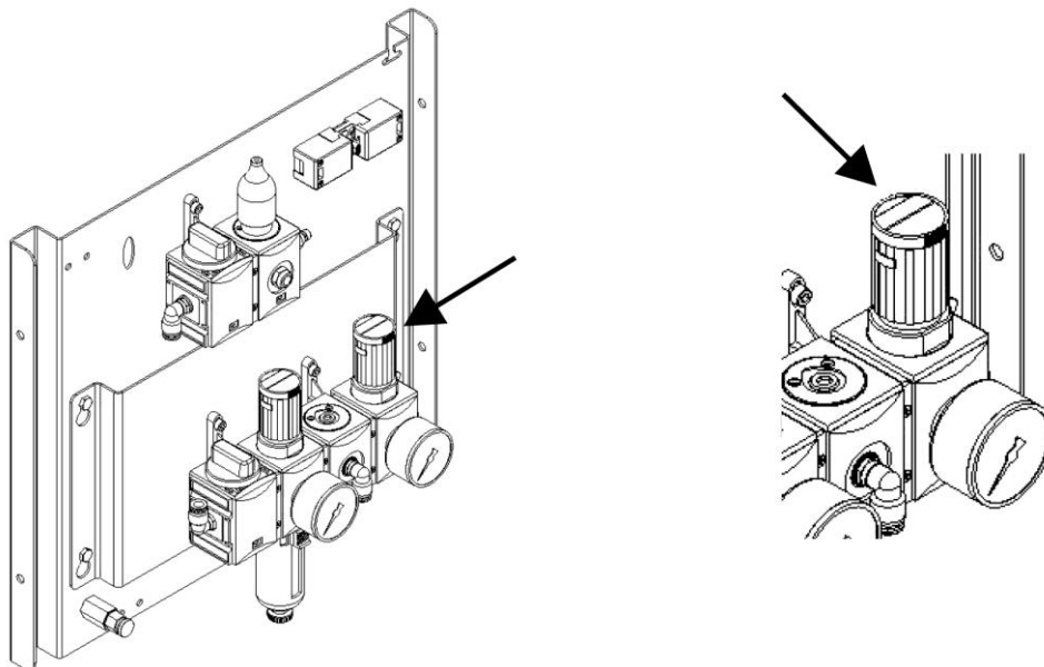
Bild 30: Ställa in trycket för lyftanordning / stoftsamlingsbehållare
