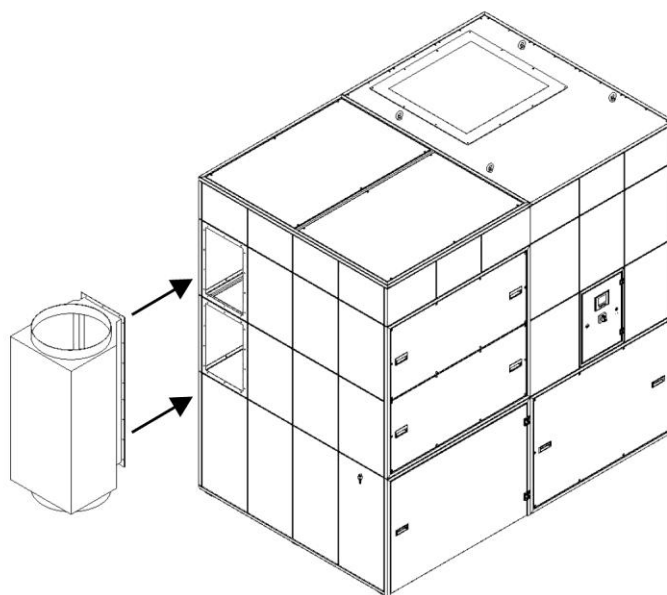
Bild 26: Montera anslutningslådan på sugsidan
