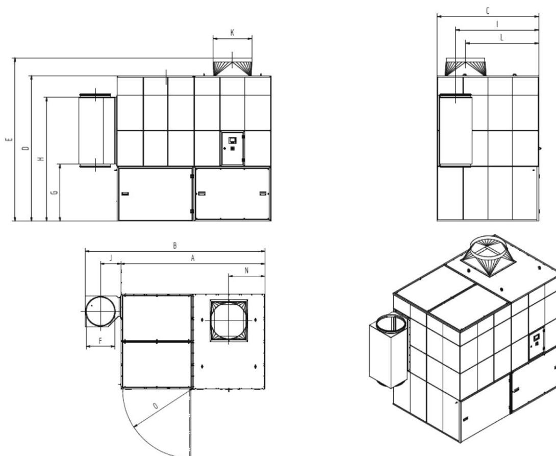
Bild 75: Måttblad 34110
