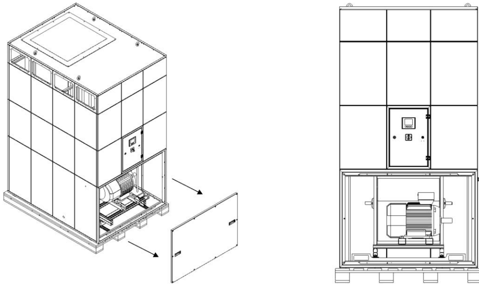
Bild 9: Fläktedel, öppna underhållsdörr
