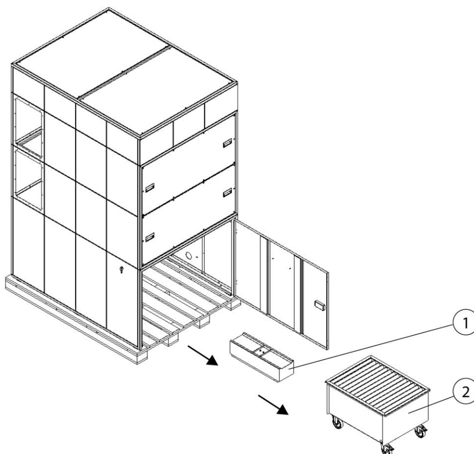
Bild 16: Ta bort stoftsamlingsbehållaren och lyftanordningen
