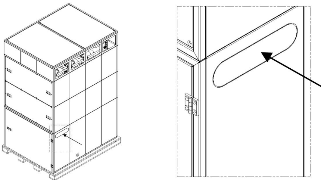
Bild 13: Långhålsplåt
