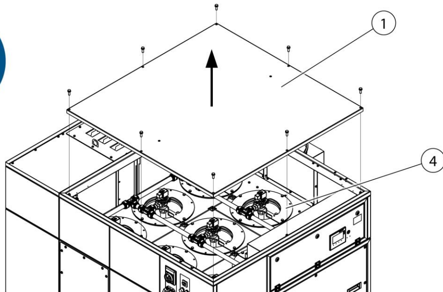
Bild 64: Filterbyte – demontera lockplåt
