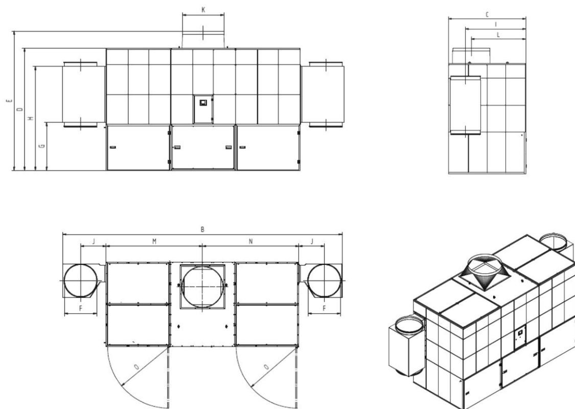
Bild 79: Måttblad 34200 + 34220
