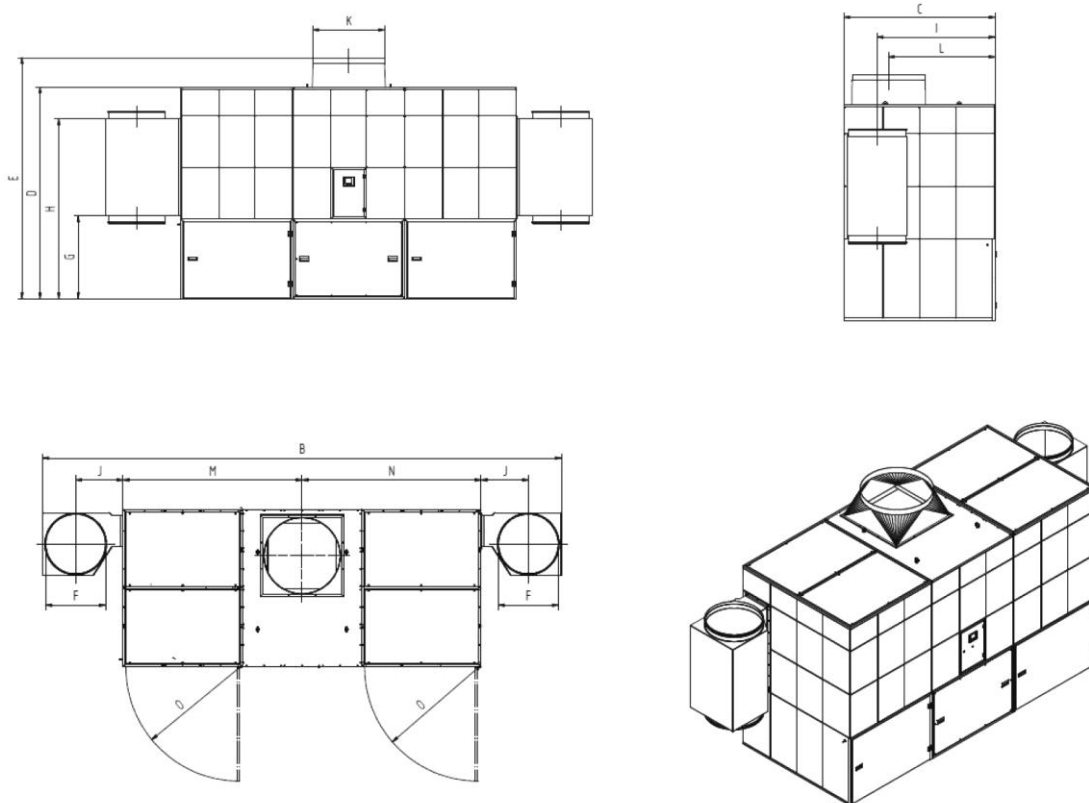
Bild 78: Måttblad 34180
