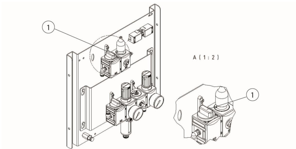
Bild 55: Tryckluftsventil stoftsamlingsbehållare
