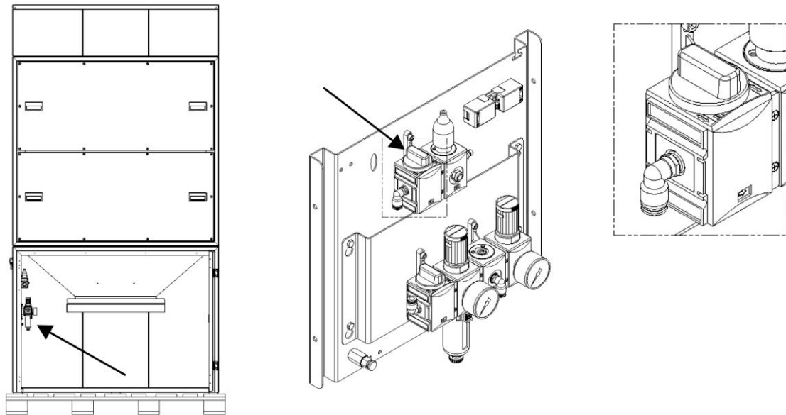
Bild 14: Sänkventil stoftsamlingsbehållare
