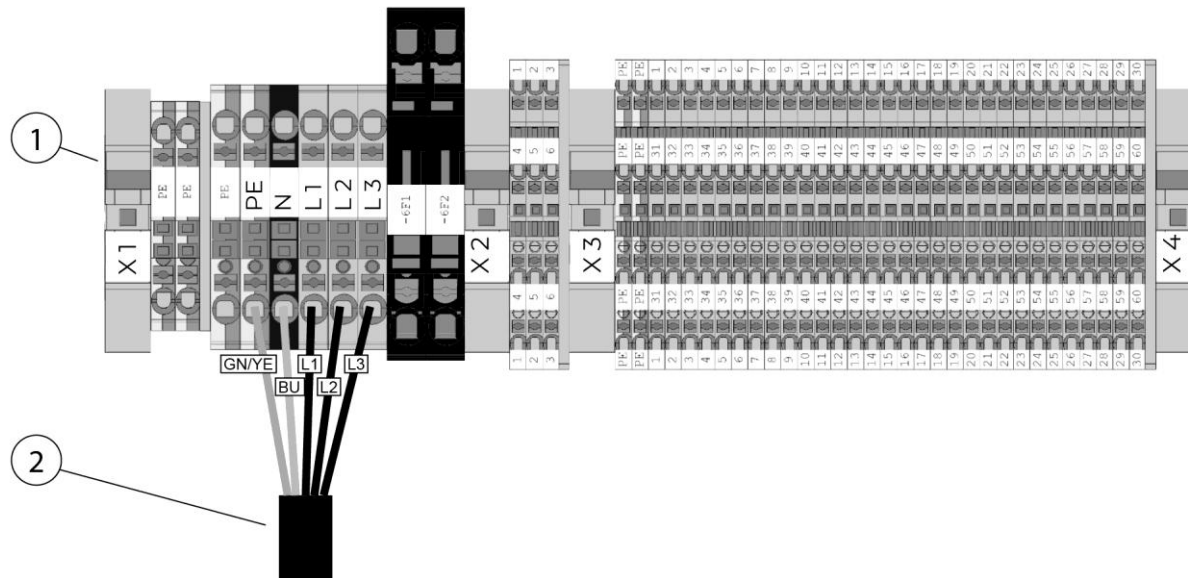
Bild 32: Anslutningsplint kopplingsskåp produkt
