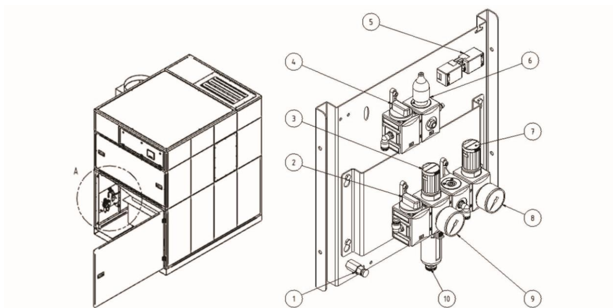
Bild 27: Tryckluftsenshet
