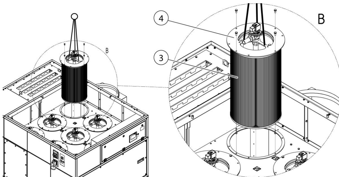
Bild 67: Filterbyte – demontera filterfäste
