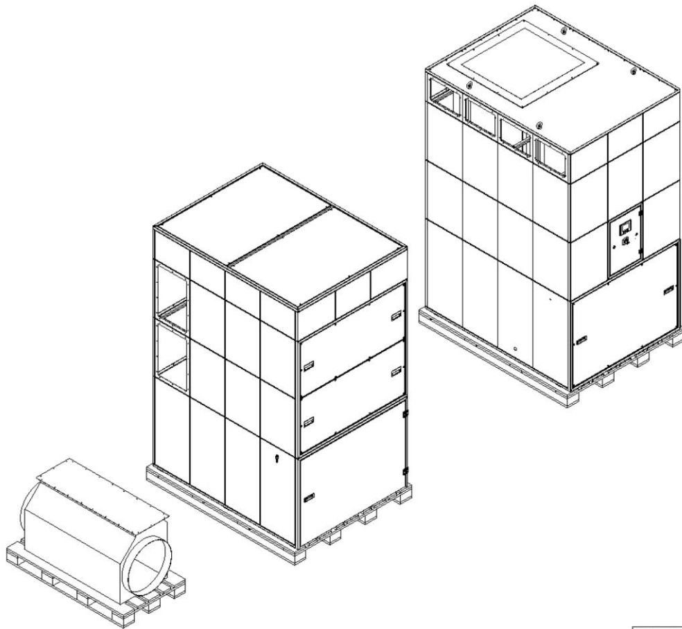
Bild 6: Leveransskick
