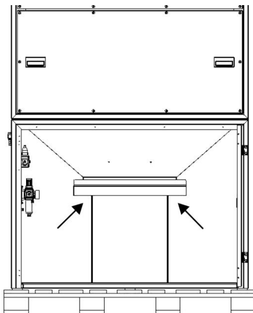
Bild 19: Lyfta filterdelen med gaffeltruck
