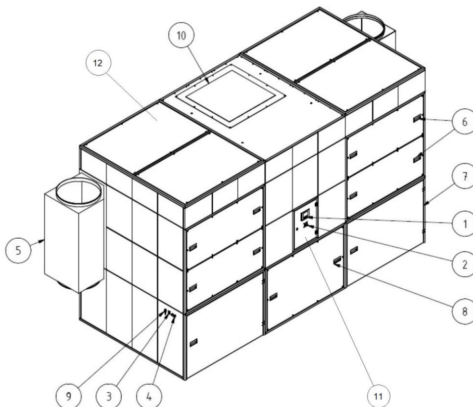
Bild 2: 34160 - 34270
