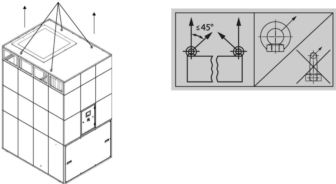
Bild 10: Lyfta fläktdelen med kran
