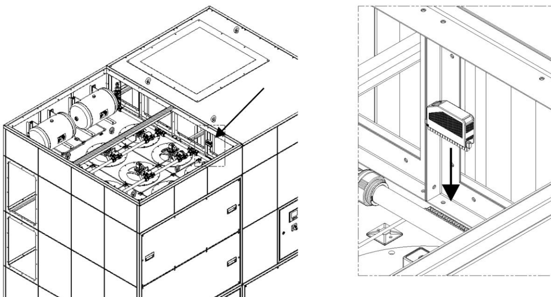
Bild 22: Montera den gröna stickkontakten
