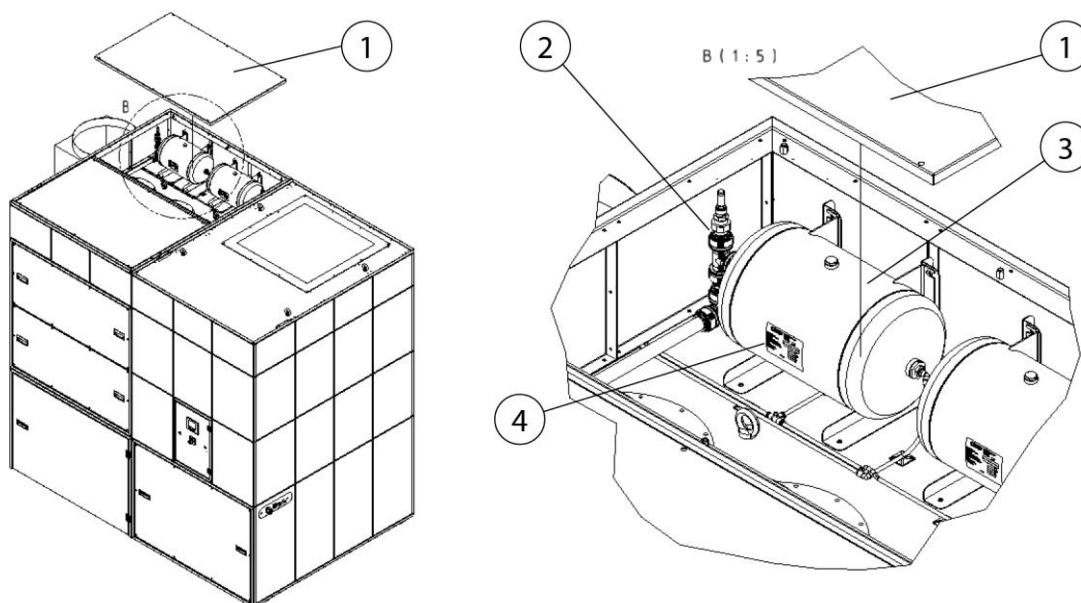
Bild 74: Åtkomst till tryckluftsbehållare + säkerhetsventil
